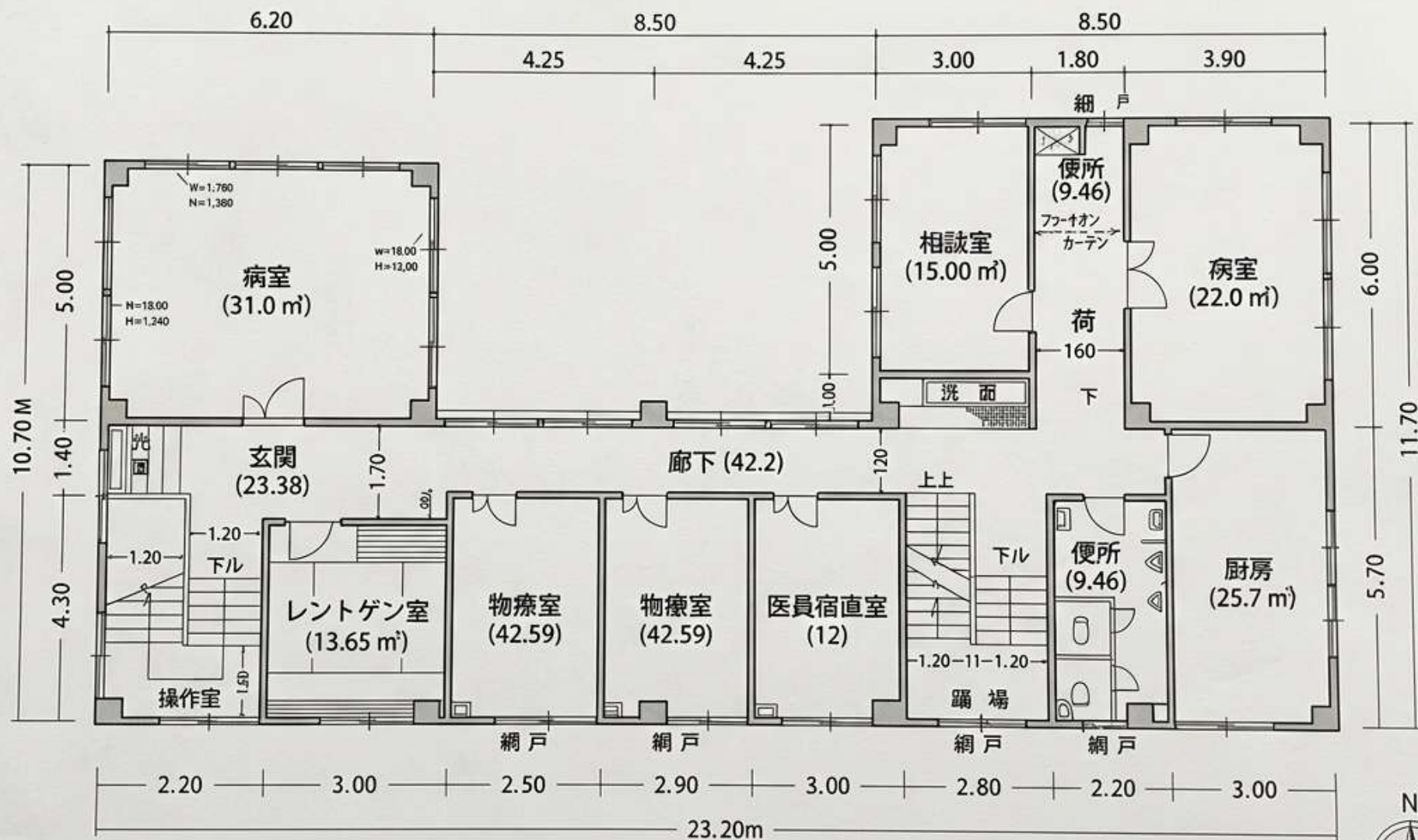
2 階平面図
