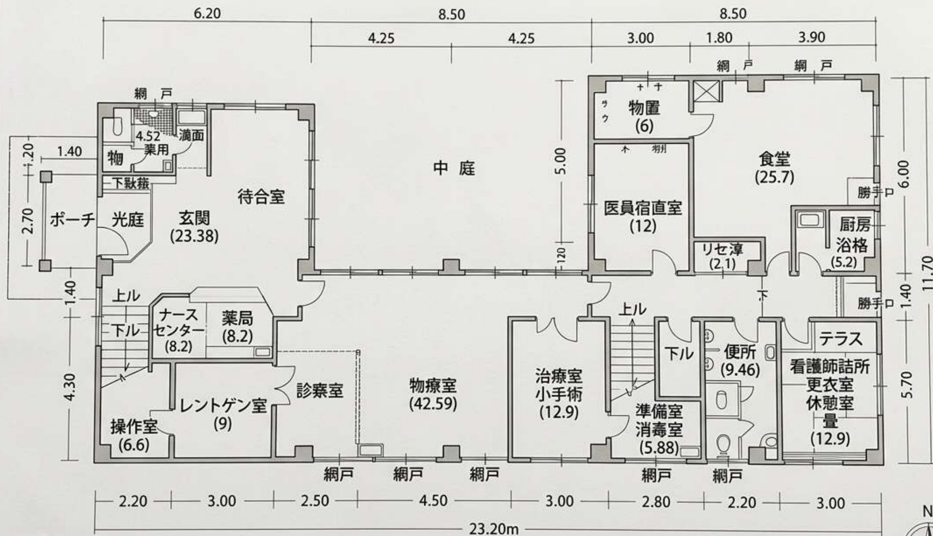
1階平面図 (1階)
