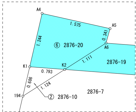
拡大図1/50
